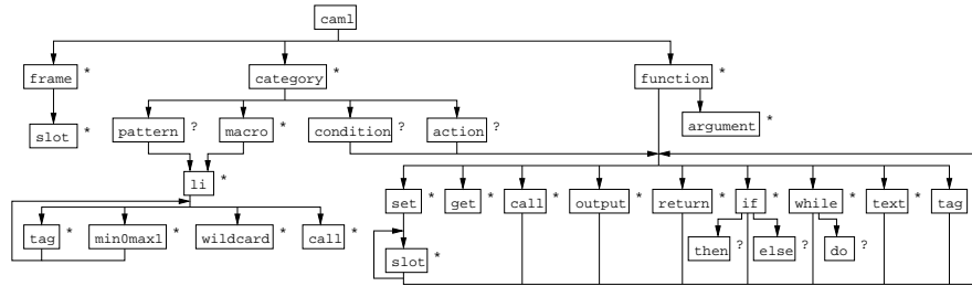
Fig. 2. CAML DTD
